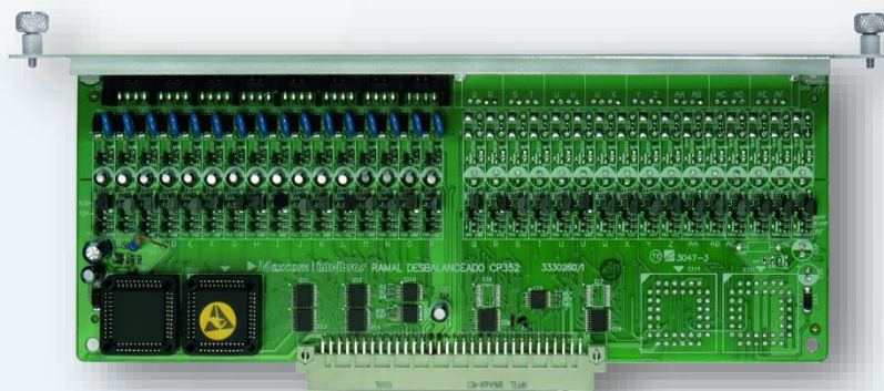
Placa de 16 Ramais Desbalanceados
