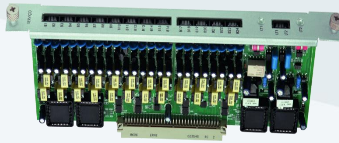
Placa de Serviço – CP 192 / CP 352
