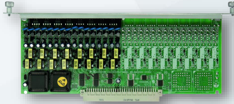
Placa de 16 Ramais Balanceados
