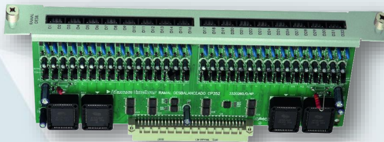
Placa de 32 Ramais Desbalanceados
