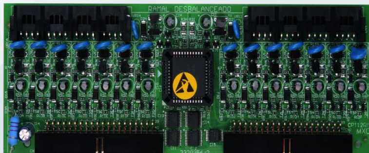
Placa de 16 Ramais Desbalanceados
